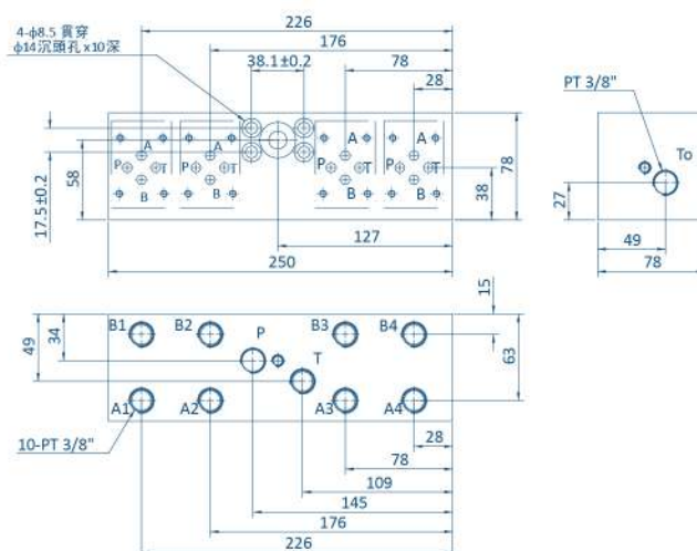
F4 (適用泵浦類型: AR柱塞泵,VD葉片泵)
