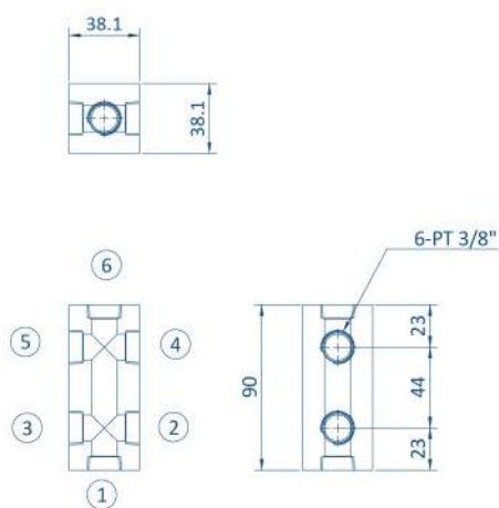
T3 (適用泵浦類型: AR / V 柱塞泵,VD葉片泵)
