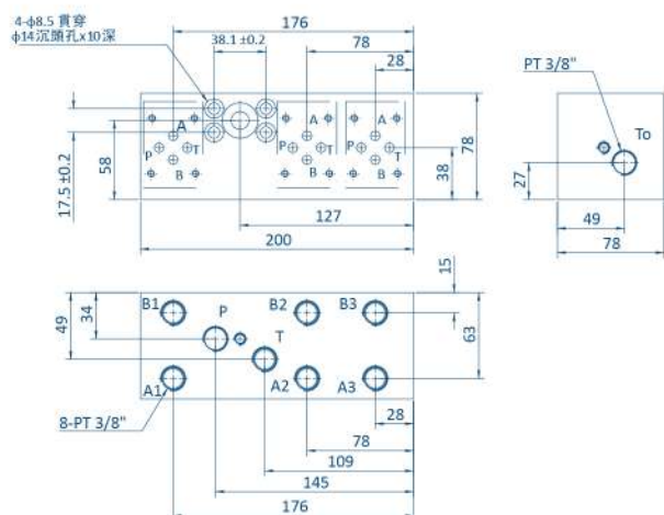
F3 (適用泵浦類型: AR柱塞泵,VD葉片泵)
