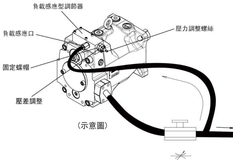
負載感應型調節器+總壓保護 HA
