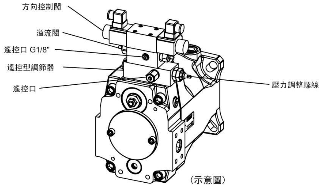
遙控型調節器+電控卸載+兩段壓力 GC
