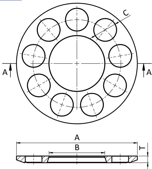
剖面圖 A-A 比例 1 : 1.2
