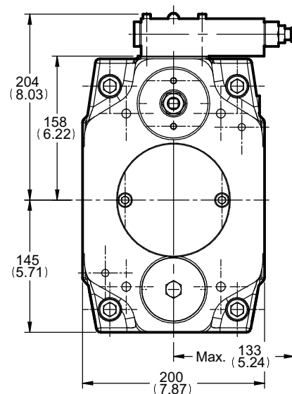
X向視圖
