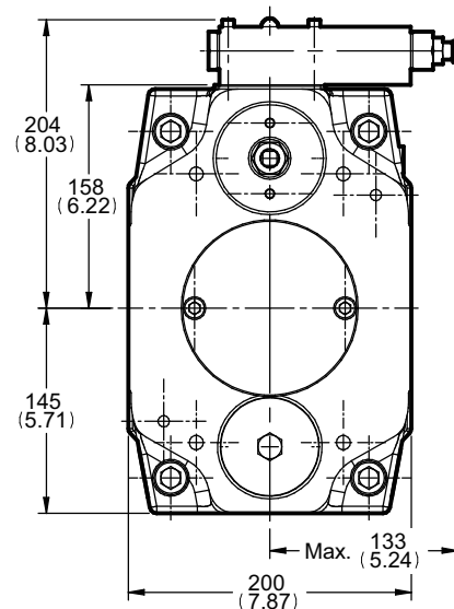
X向視圖
